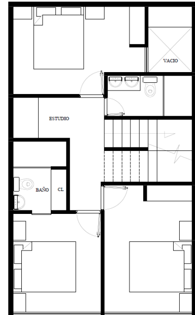
PL PLANTA ARQUITECTÓNICA 2 NIVEL ESCALA 1/75
