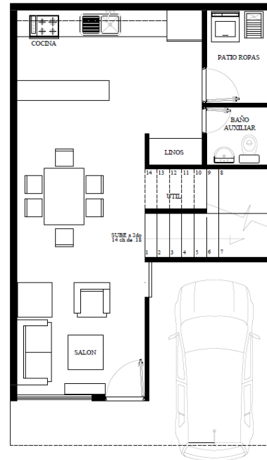
PL PLANTA ARQUITECTÓNICA 1 NIVEL ESCALA 1/75
